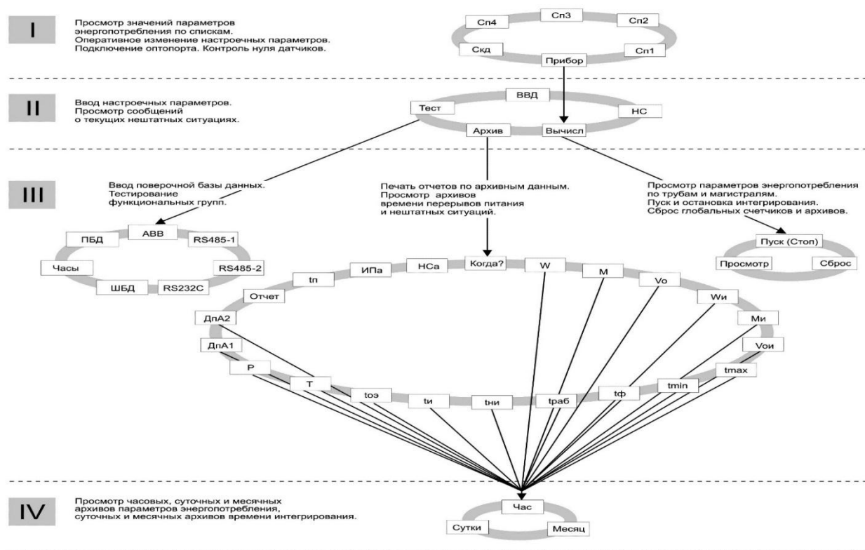
Рисунок 6.1 – Структура меню
