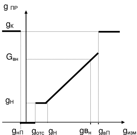
Рисунок 2.5 – Преобразование измеренных значений массового расхода
