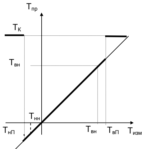
Рисунок 2.6 Преобразование измеренных значений температуры
