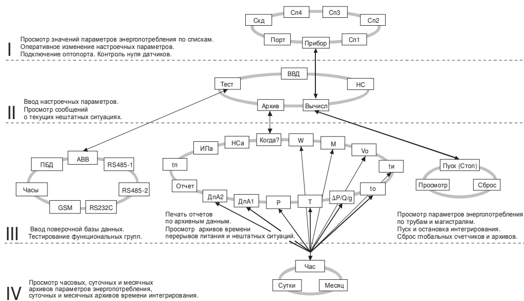
Рисунок 5.1 – Структура меню
