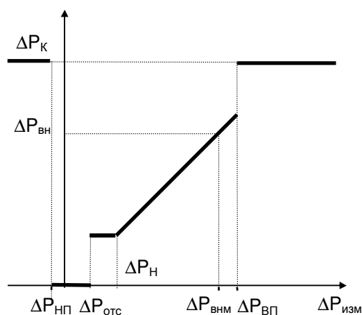
Рисунок 2.3 – Преобразование измеренных значений перепада давления
