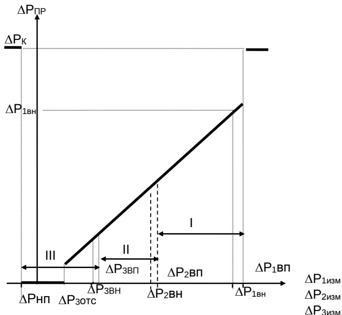
Рисунок 4.6 – Преобразование значений перепада давления, измеренных тремя датчиками
