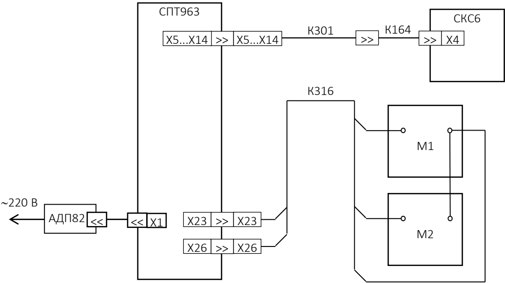
Рисунок 11.2 – Схема проверки. M1, M2 – магазин сопротивлений Р4831
