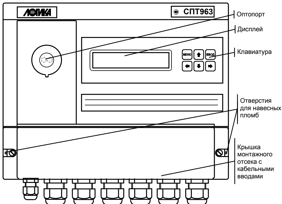
Рисунок 3.1 – Вид спереди
