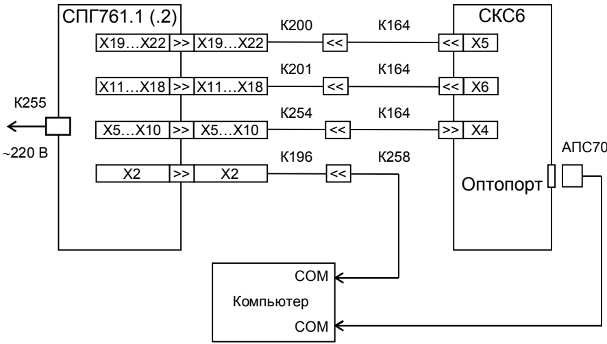
Рисунок 9.1 Схема проверки
