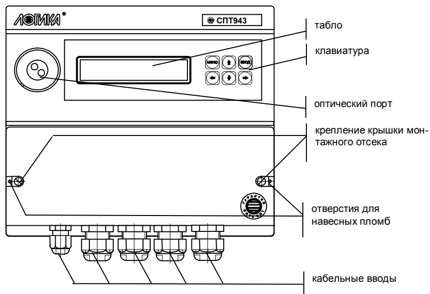
Рисунок 3.1 – Вид спереди
