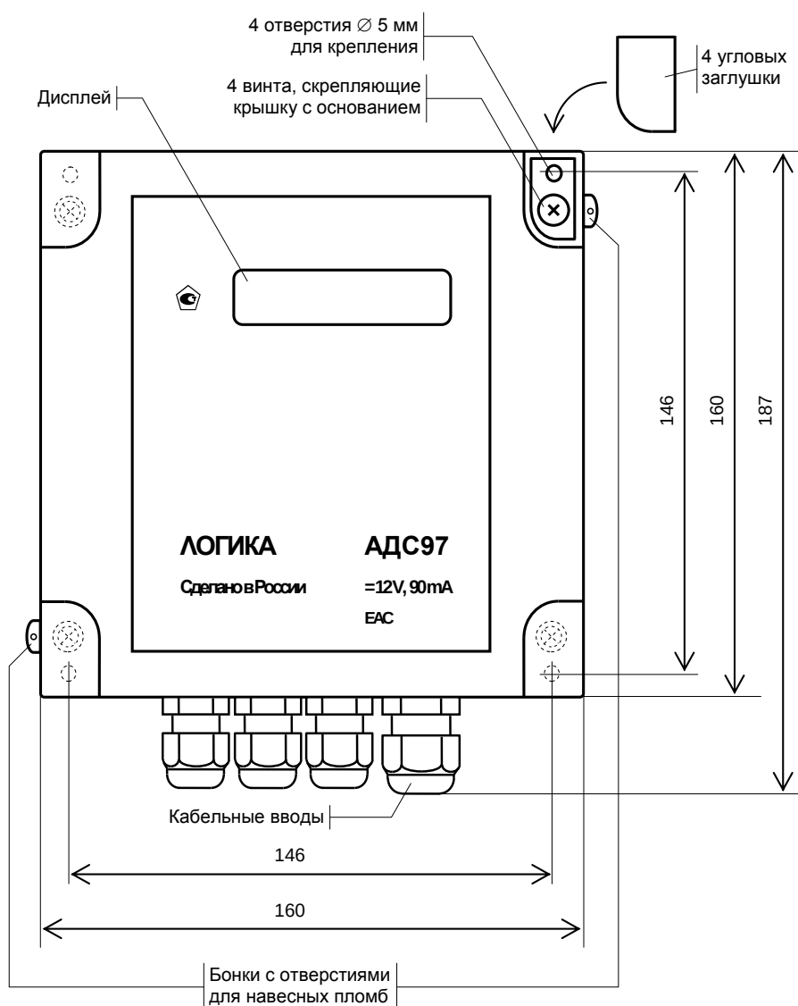
Рисунок 3.1– Вид спереди
