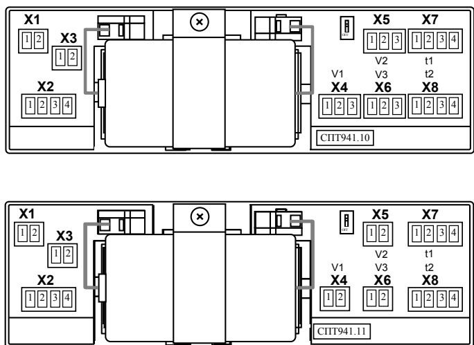
Рисунок 10.1 – Размещение гнезд для подключения внешних цепей
